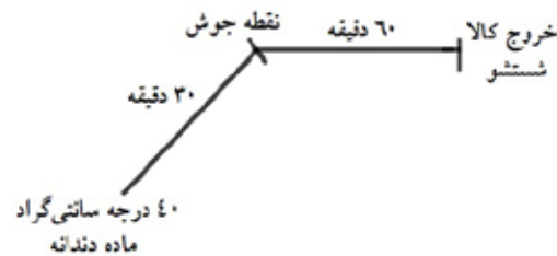
تصویر ۶: گراف دندان‌دادن کالای پشمی (مأخذ: نگارندگان)
