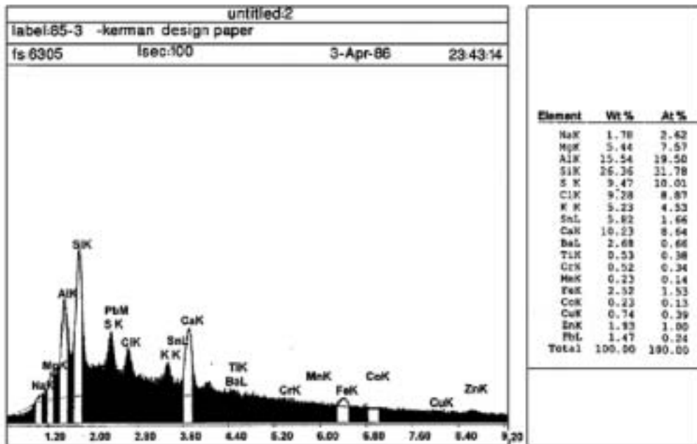
شکل ۱۰: آنالیز عنصری SEM پرکننده‌ها و پوشاننده‌های کاغذ نقشه قالی بدون تکیه گاه کرمان
