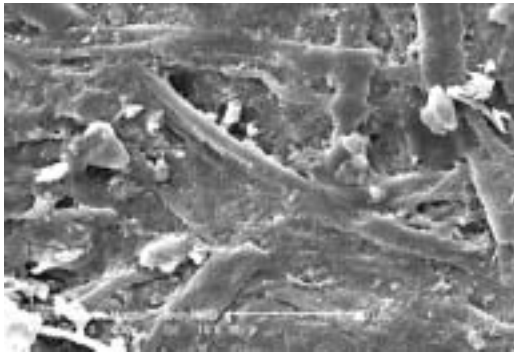
شکل ۱۳: عکس میکروسکوپ الکترونی SEM الیاف، پرکننده‌ها و پوشاننده‌های کاغذ نقشه قالی اصفهان با بزرگ‌نمایی ۴۰۰x
