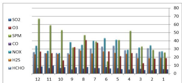
نمودار ۲- آلاینده‌های موجود در فصل تابستان در سالن موزه‌ی فرش (نگارنده، ۱۳۹۵)
