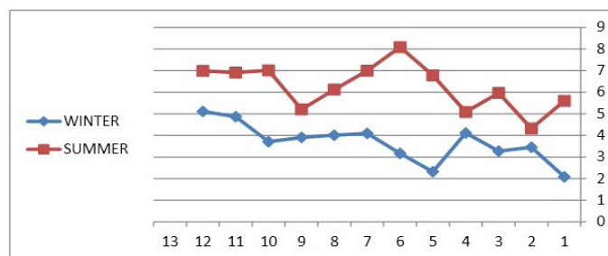
نمودار ۶- سنجش CO (ppb) در زمستان و تابستان موزه‌ی فرش ایران (نگارنده، ۱۳۹۵)
